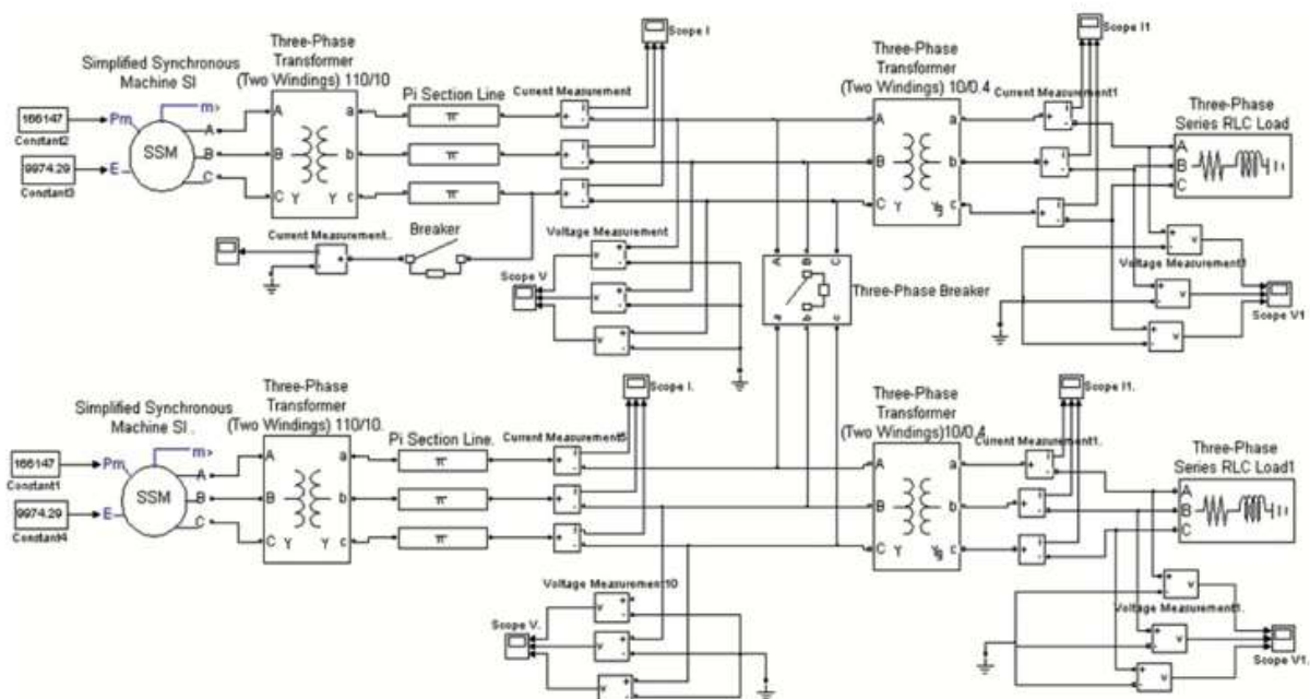
Рисунок 2 – Имитационная модель участка электрической сети
