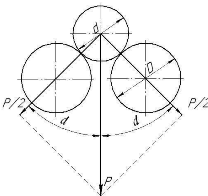
Рисунок 2 – Схема статического уравнивания изделия на направляющих роликах
