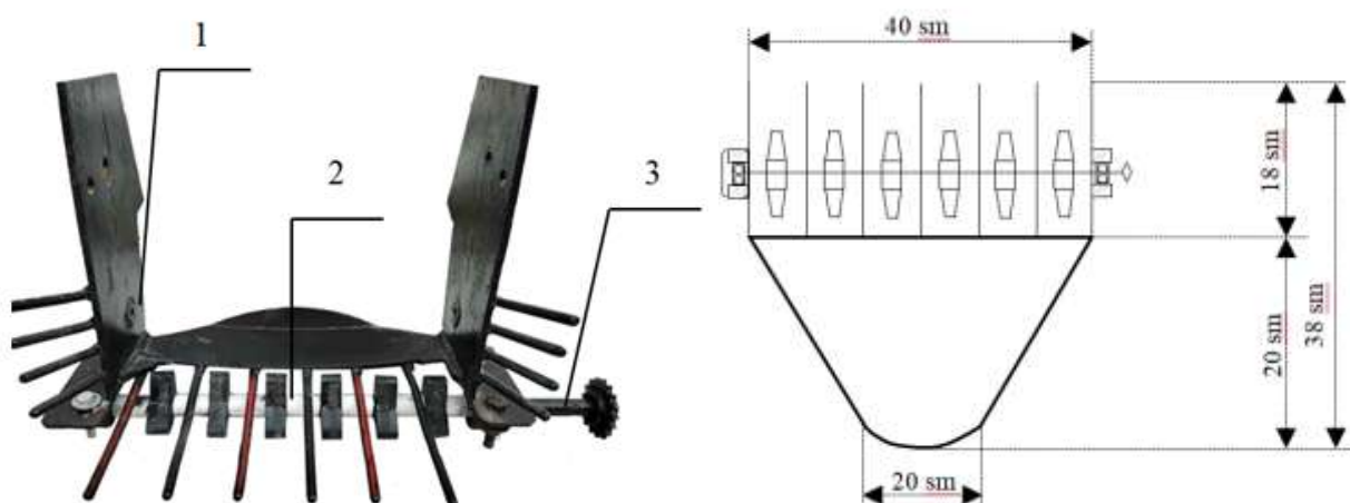
Рисунок 3 – Лемех с пальцевым ротором
