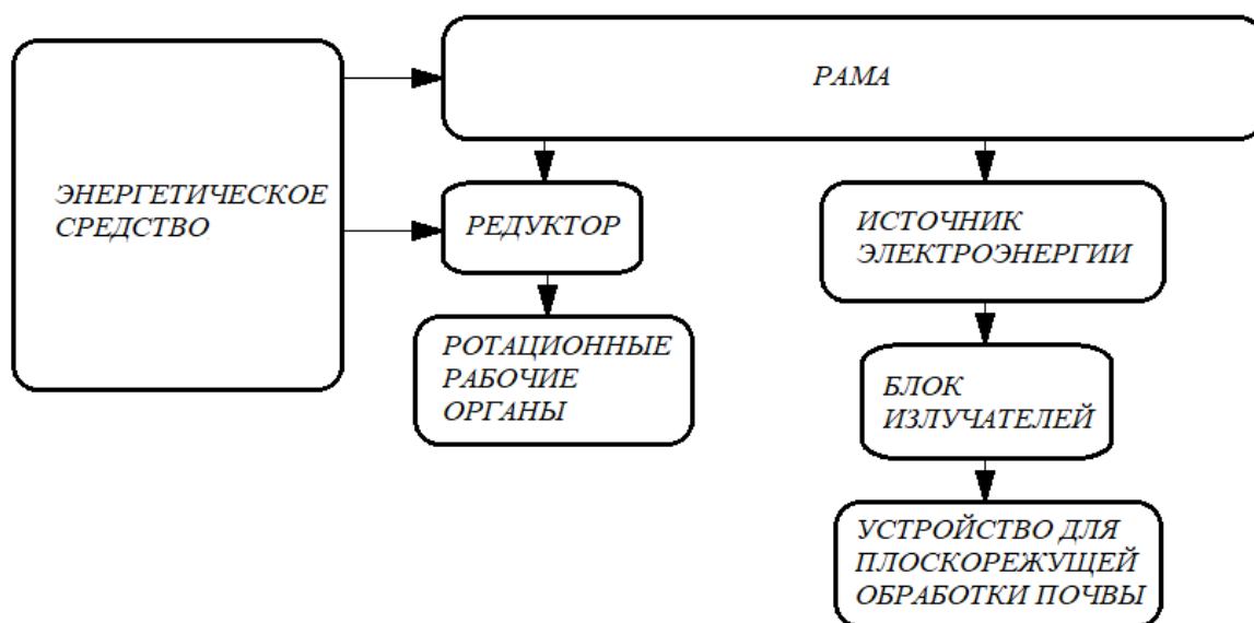
Рисунок 8 – Функциональная схема прицепной машины для обеззараживания почвы
