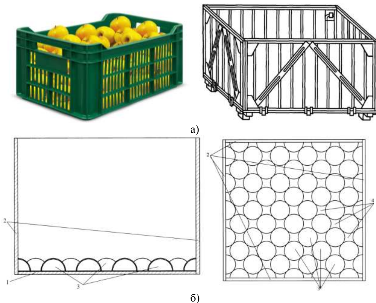
а – вид сбоку; б – вид сверху; 1 – дно; 2 – стенки контейнера; 3 – упругие выступы; 4 – ячейки, образованные четырьмя Рисунок 4 – Универсальные пластмассовые ящики
