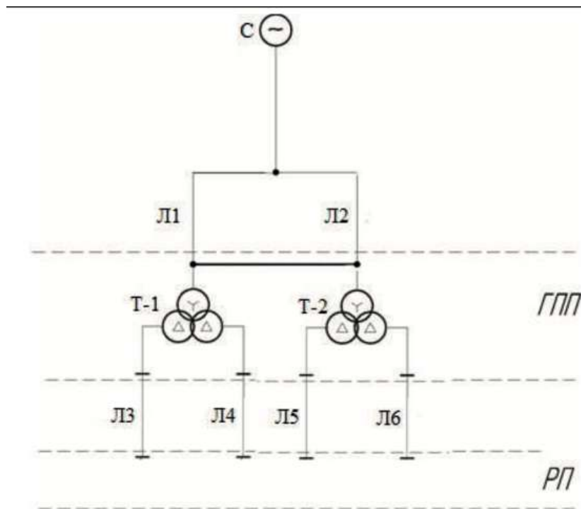
Рисунок 1 – Упрощенная электрическая схема участка городской сети [4]
