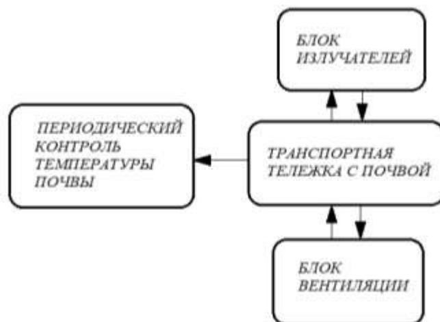
Рисунок 1 – Структурная схема стационарной машины для обеззараживания почвы
