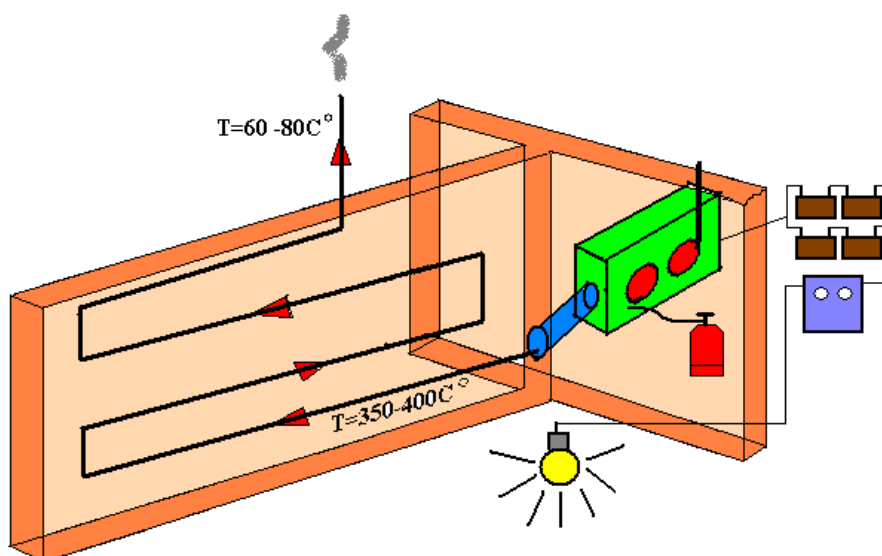
Рисунок 1 – Печь с системой водяного отопления
