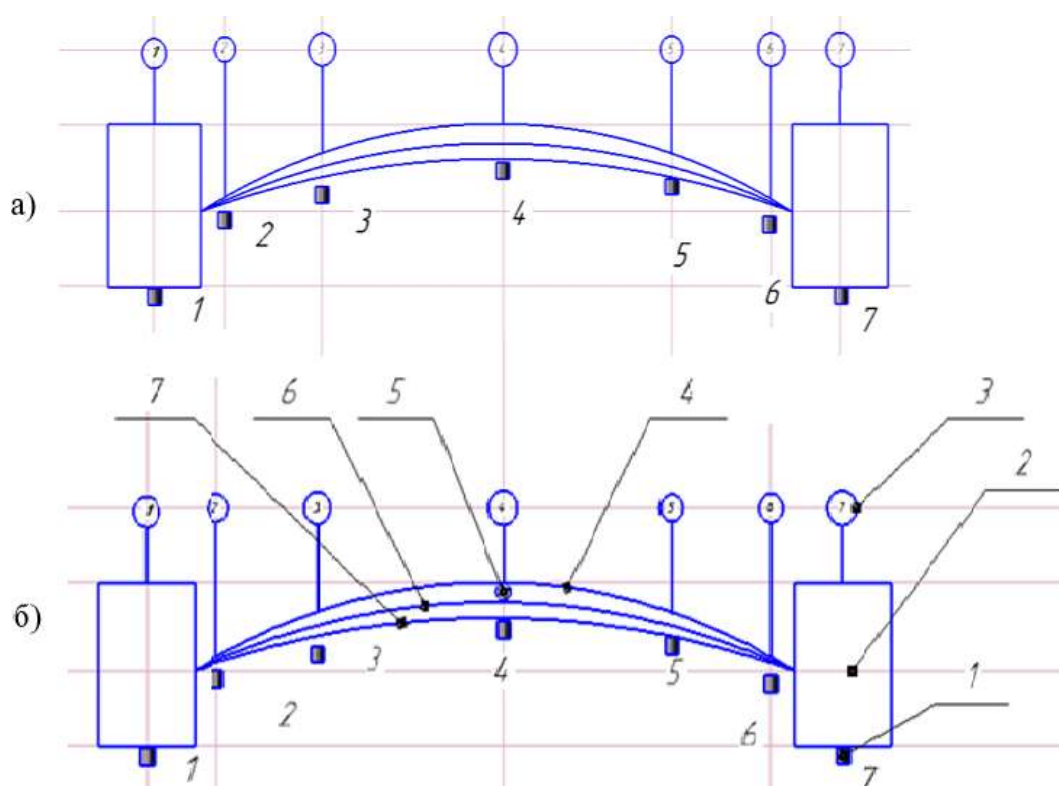
а) статически неопределимая конструкция СБФО;
