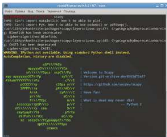
Рисунок 1 – Интерфейс Scaru
