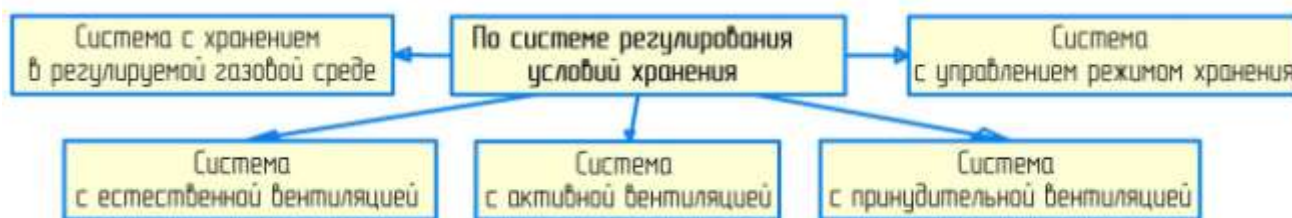
Рисунок 4 – Схема деления картофелехранилищ по системам регулирования условий хранения
