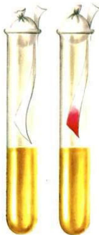
Рисунок 56 - Определение индола.
