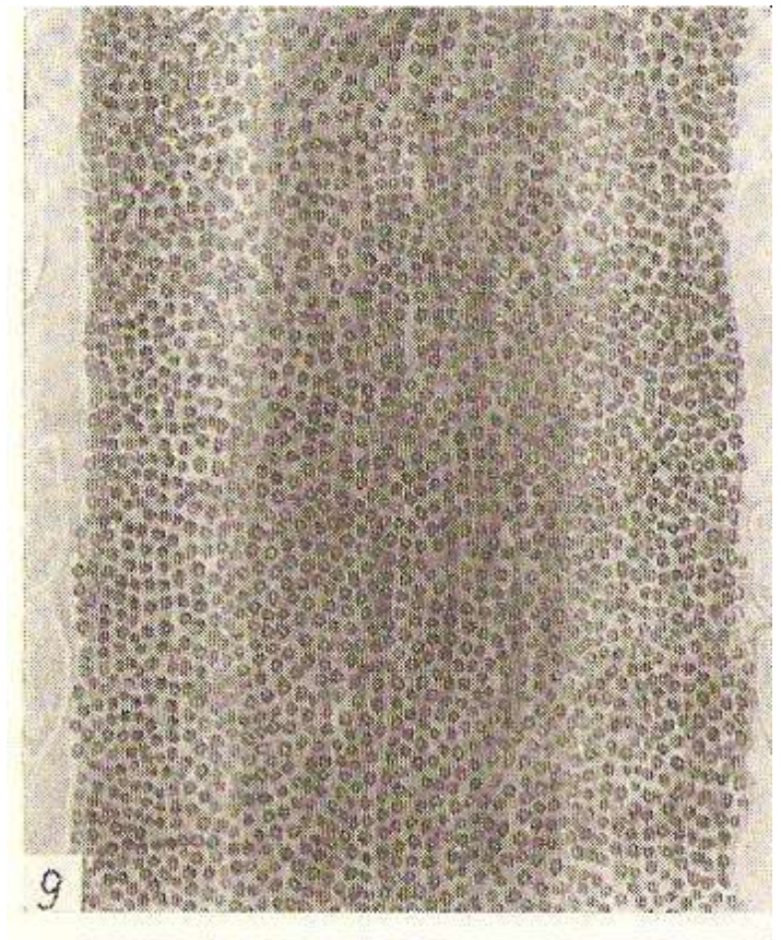
Рисунок 140 - Возбудитель микроспории.
