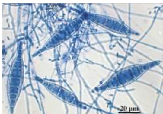
Рисунок 32 - Microsporum canis.
