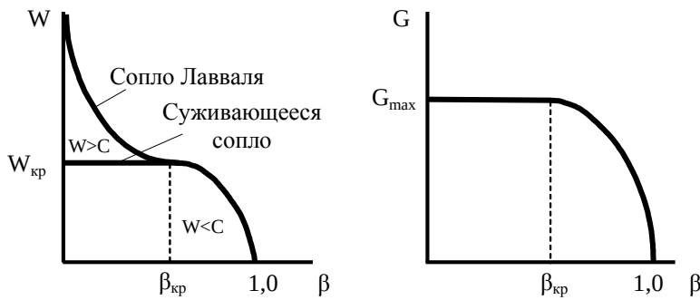
Рис. 3. Изменение скорости истечения и расхода газа через суживающееся сопло и сопло Лавалья от отношения давлений.
