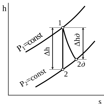
Рис. 4. Изобэнтропийный и действительный процессы истечения газа в sh - диаграмме
