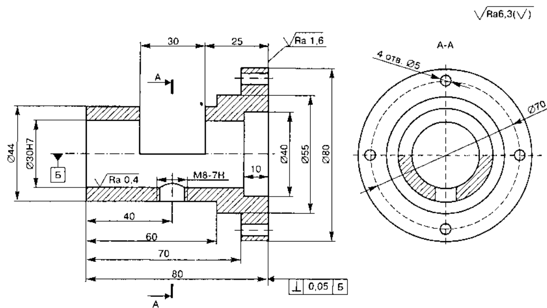
Рисунок 8 - Фланец
