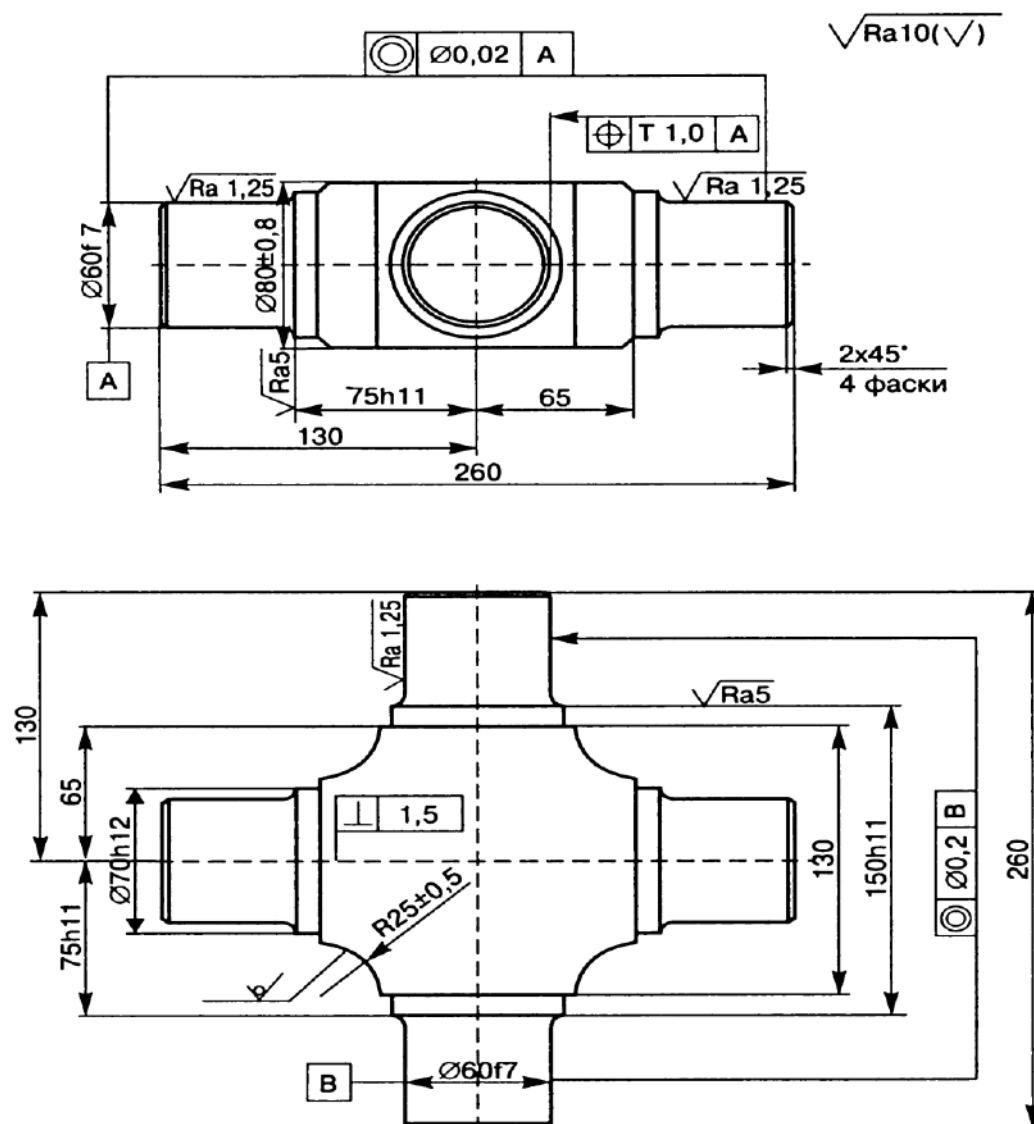
Рисунок 4 - Крестовина
