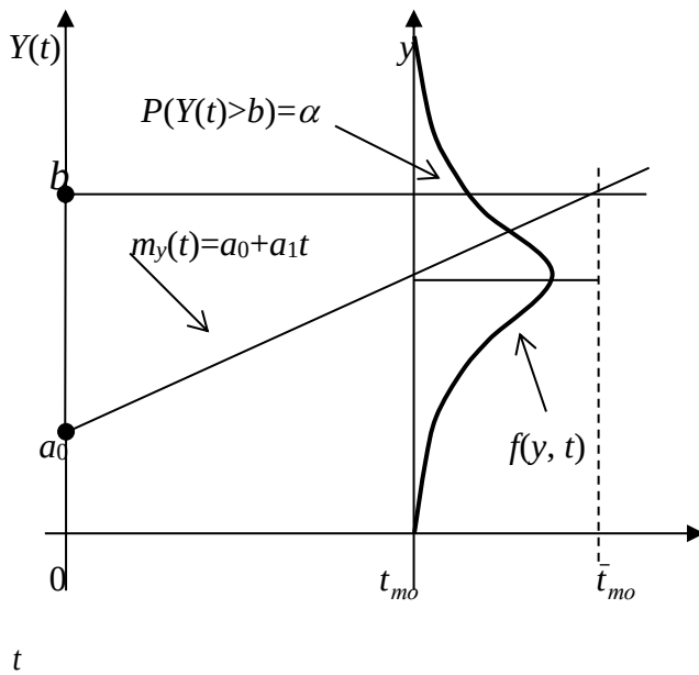
Рис. 2. Вероятностная оценка предельной наработки t = t_{mo} автомобиля при заданном риске \alpha превышения техническим параметром Y(t) как случайной функцией предельно допустимого значения b . Игнорирование вероятностного поведения Y(t) даёт завышенное значение предельной наработки t = \bar{t}_{mo} > t_{mo} .
