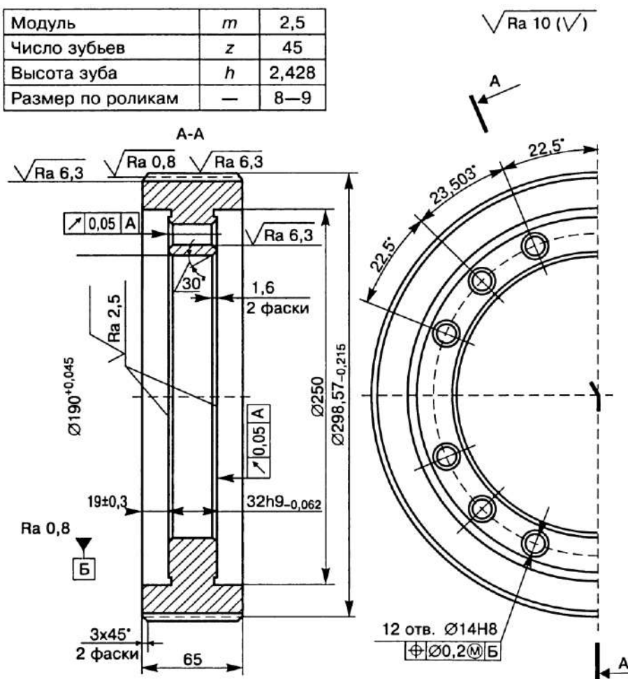
Рисунок 5 - Шестерня
