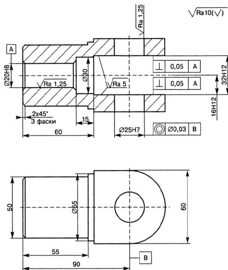
Рисунок 3- Серьга
