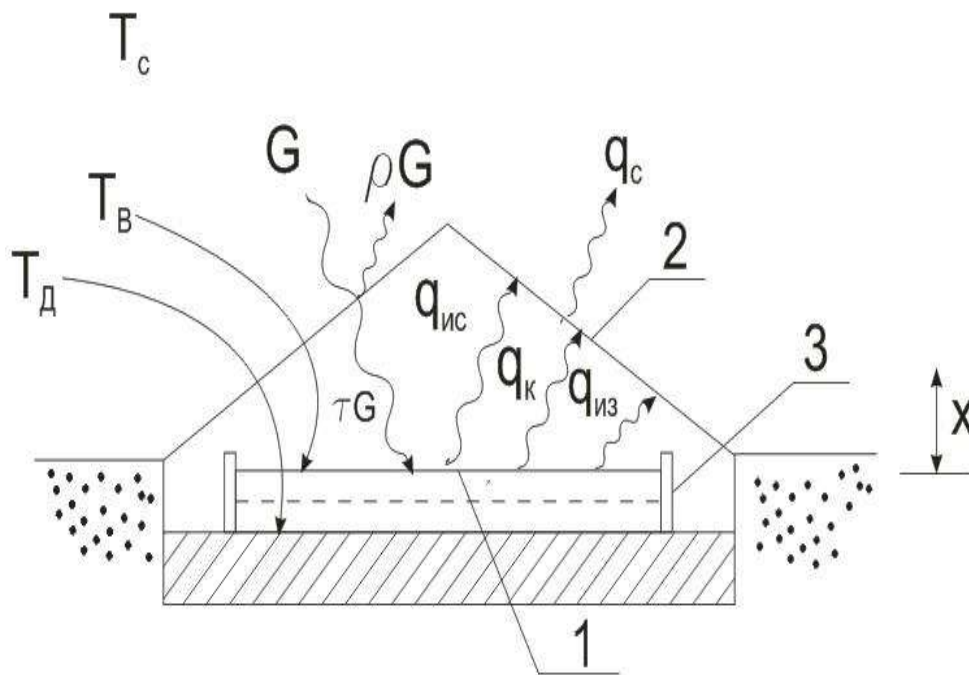
Рисунок 9.1. - Потокн тепла в солнечном днстнлляторе.
