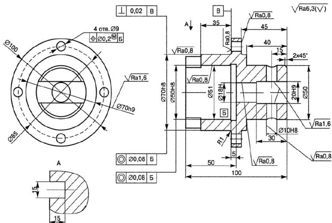
Рисунок 9 - Крышка
