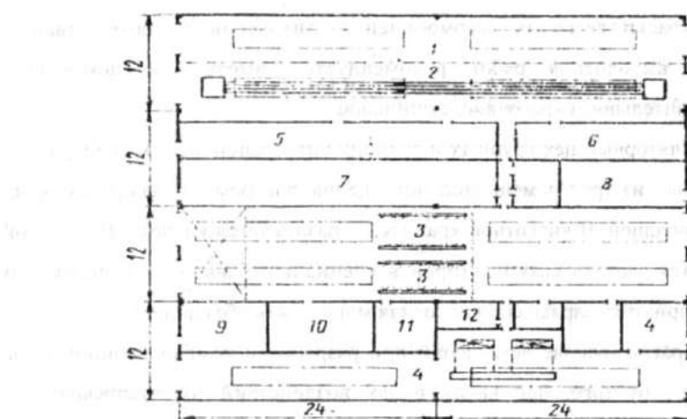
Рис. 7.11. Компоновочный план вспомогательного корпуса АТП. 1-Пост общей диагностики; 2-Пост перестановки колес; 3-Поточные линии ЕО; 4-Малярная; 5-Склад шин; 6-Шинномонтажная; 7-Бытовые помещения; 8-Компрессорная; 9-Трансформаторная; 10-Такелажная; 11-Комната мойщиков; 12-Электрощитовая.
