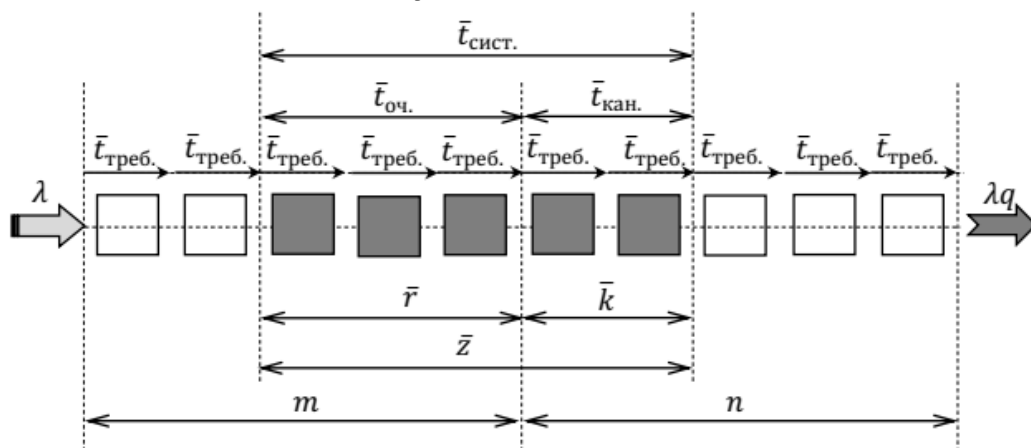
Рис. 9. Схема усреднённой в вечности СМО.
