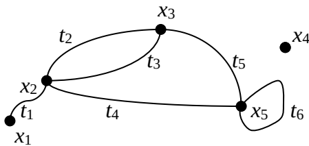
Рис.3. Неориентированный граф с вершинами X = \{x_1, x_2, x_3, x_4, x_5\} и рёбрами T = \{t_1, t_2, t_3, t_4, t_5, t_6\} . При этом t_2, t_3 – кратные рёбра, t_6 – петля, x_4 – изолированная вершина.
