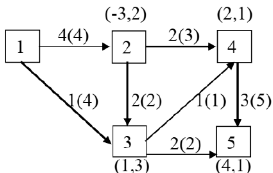
Рис. 7. Метки и увеличивающий путь P_2: 1 \rightarrow 3 \rightarrow 2 \rightarrow 4 \rightarrow 5 этапа 2. Поток можно увеличить на величину \delta=1 .
