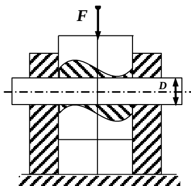
Рисунок 4. Обойма для испытания пластичного материала на двойной срез.
