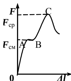
Рисунок 3. Диаграмма среза
