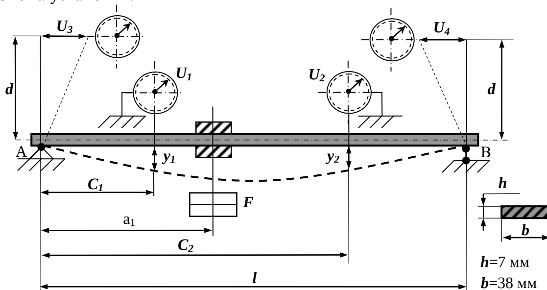
Рисунок 1. Двухопорная балка.
