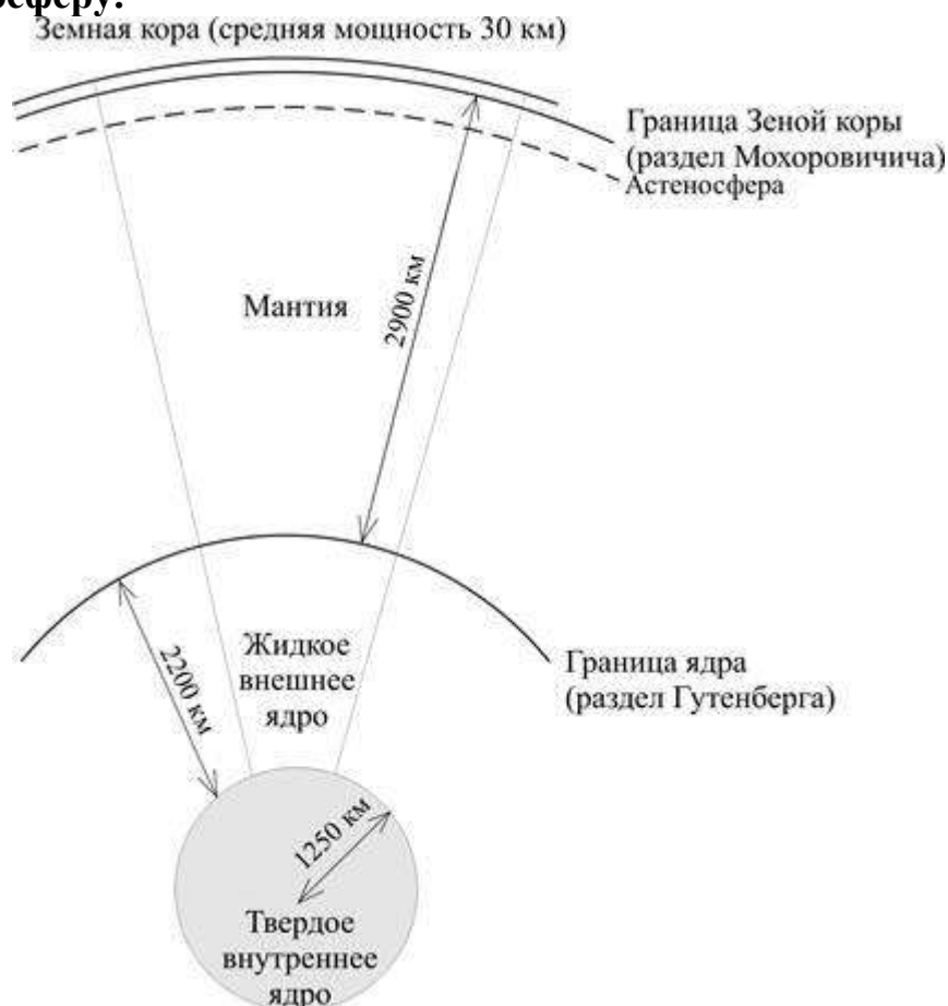
Рис. 1 Внутреннее строение Земли
