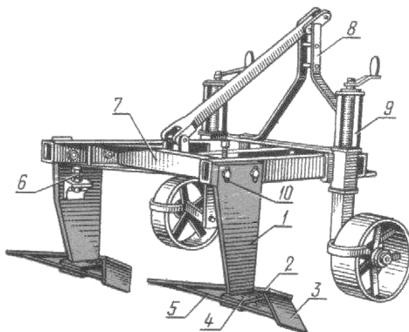
Рис. 4. Культиватор-плоскорез-глубокорыхлитель КПГ-250А: 1-стойка; 2- долото; 3- лемех; 4- пятка; 5- башмак; 6- винт; 7- рама; 8- навеска; 9- винтовой механизм; 10- овальное отверстие.
