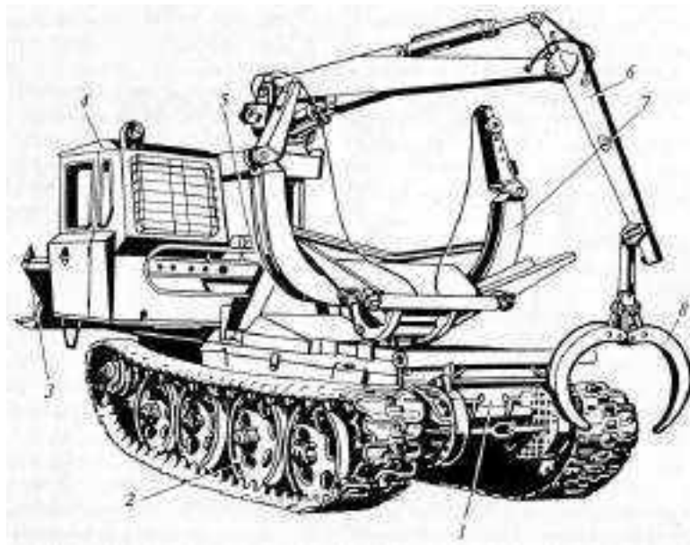
Рис. 4. Трактор ТБ-1А:
