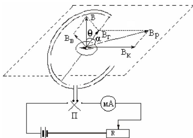
Рис.3 Схема установки
