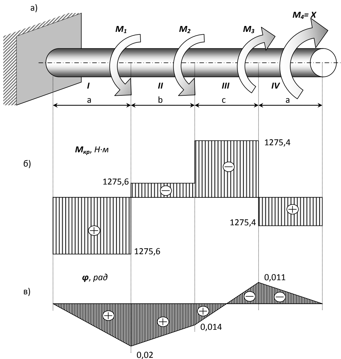
а) расчетная схема б) эпюра M_{кр}, H \cdot m ; в) эпюра \varphi, рад
