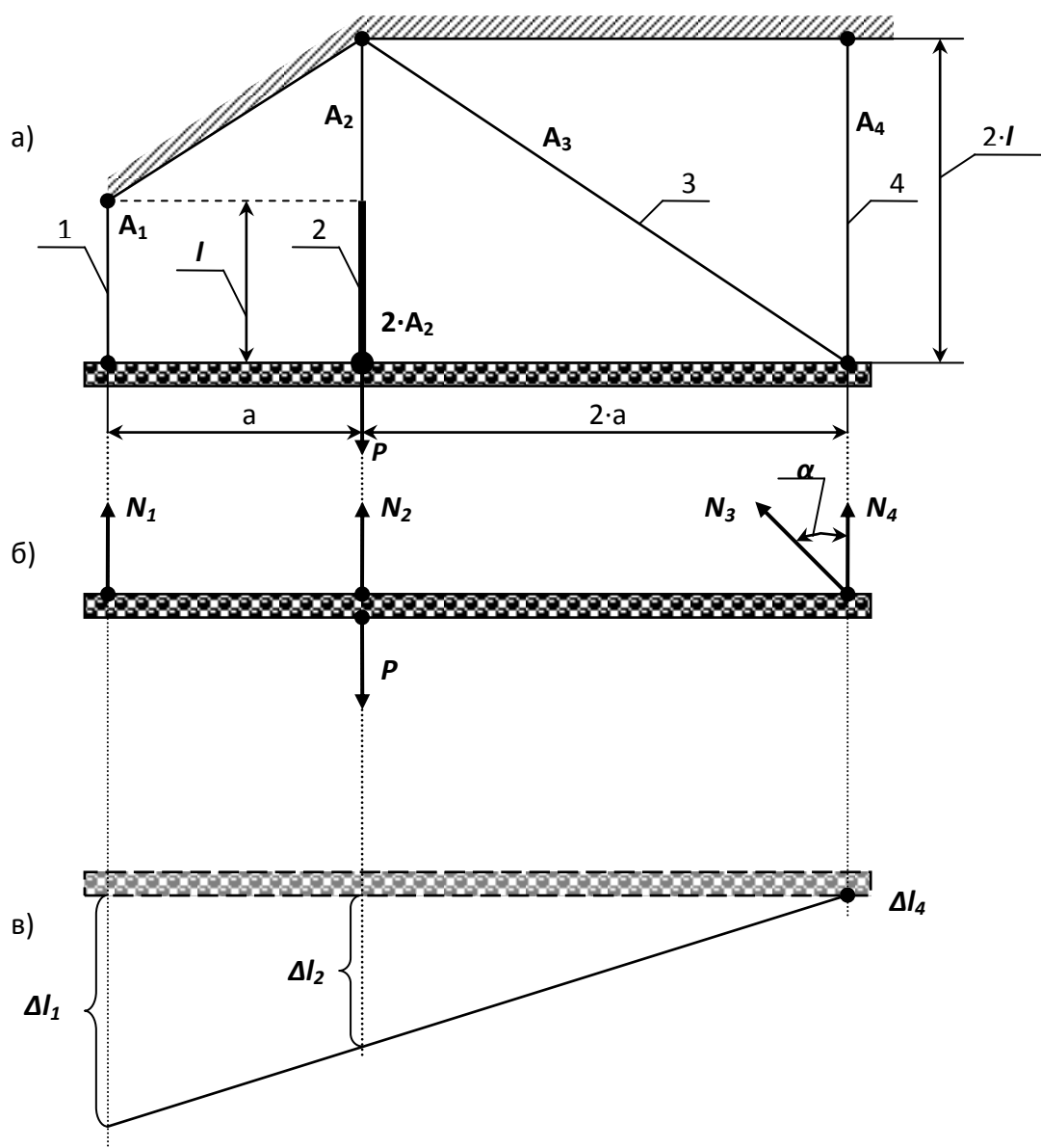
Рисунок 3.3 – Стержневая система.
