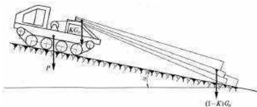
Рис. 1. Схема для расчета рейсовой нагрузки трелевочного трактора Из уравнения равномерного движения трактора с пачкой
