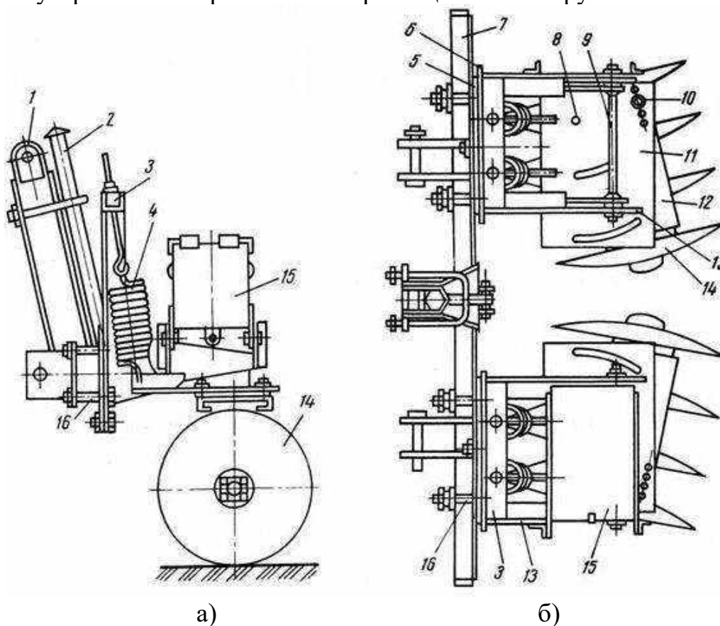
Рис.7. Культиватор лесной бороздной КЛБ-1,7:
