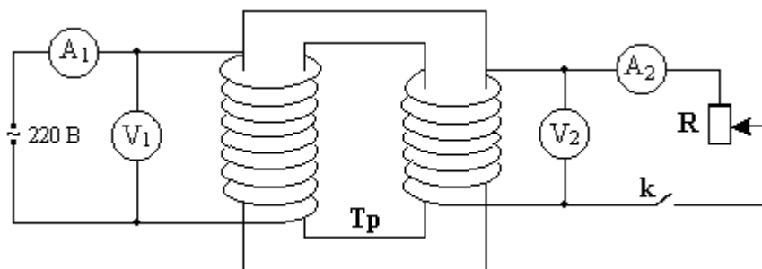
Рис.1 Схема подключения трансформатора
