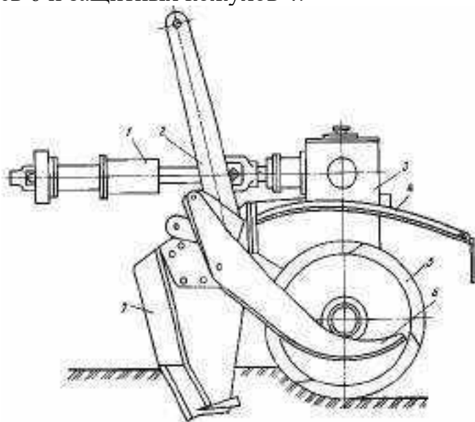
Рис. 6. Фреза лесная шнековая ФЛШ-1,2:
