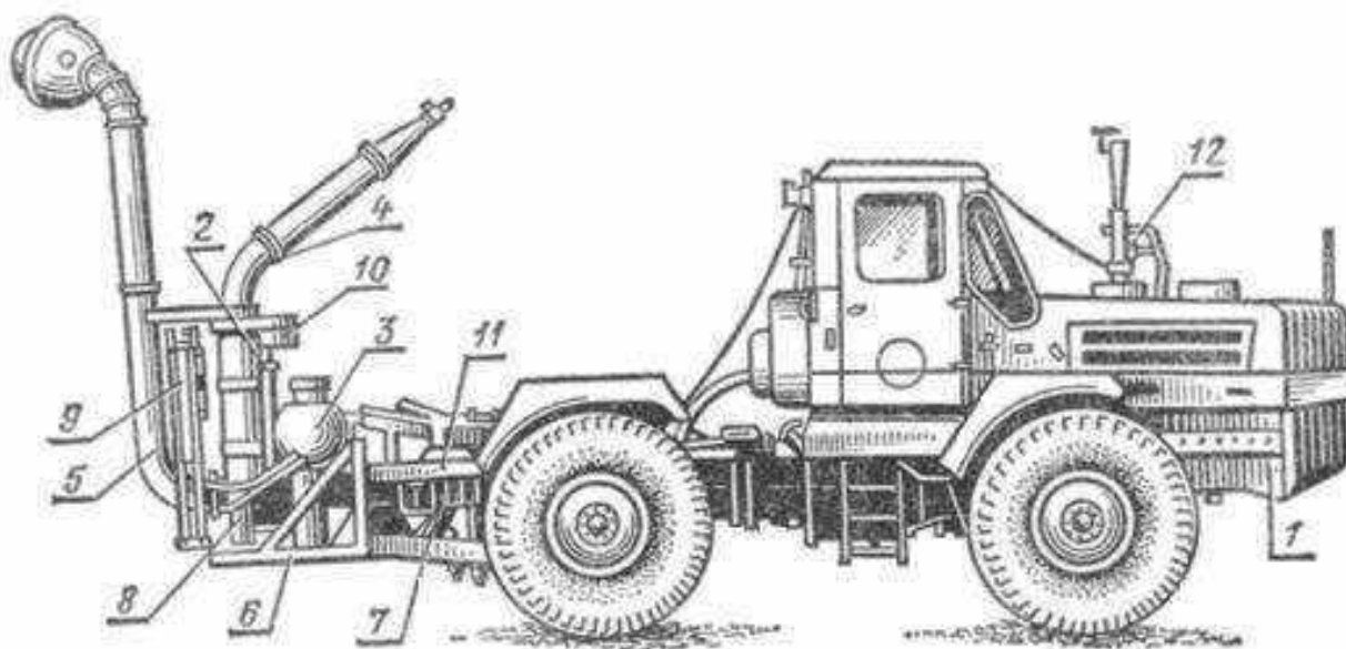
Рис. 19. Дождеватель дальнеструйный навесной ДДН-100:
