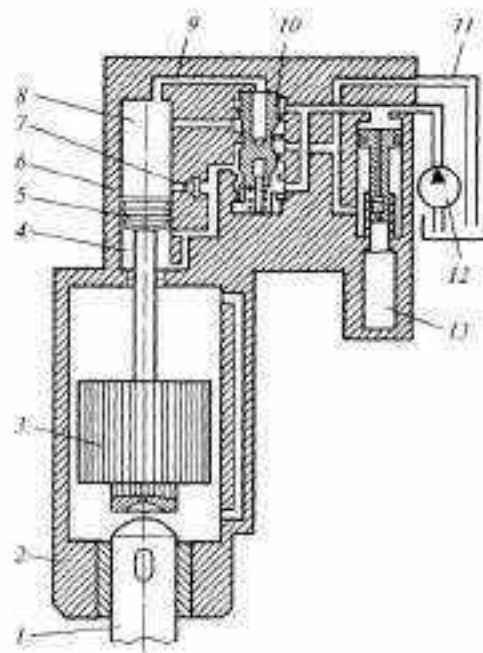
Рисунок 15. Принципиальная схема гидромолота с гидроаккумулятором
