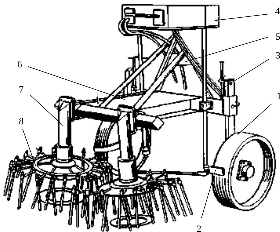
Рис. 8. Культиватор ротационный лесной КРЛ-1:
