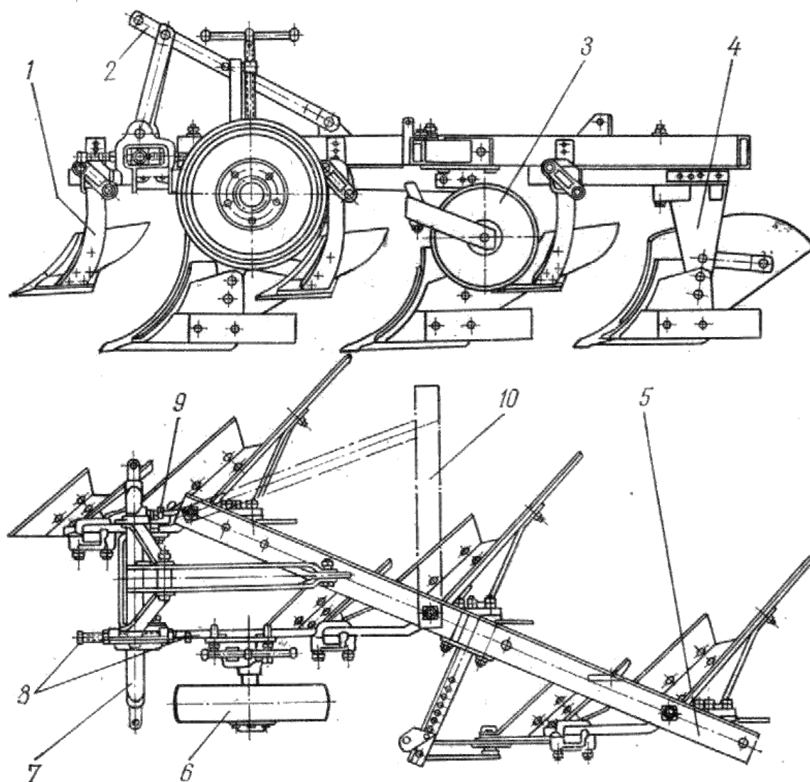
Рис. 3. Плуг лемешной навесной ПЛН-3-35:
