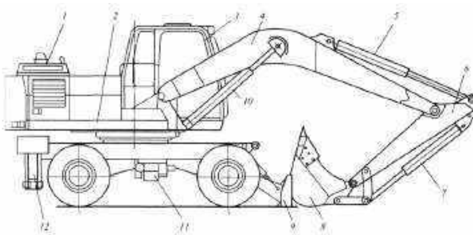
Рисунок 18. Одноковшовый полноповоротный пневмоколесный экскаватор ЕК-18:
