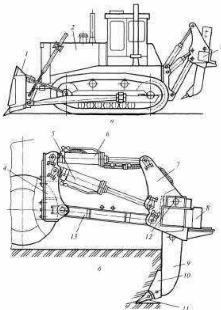
Рис. 4.12. Бульдозер-рыхлитель на базе трактора Т-25.01;
