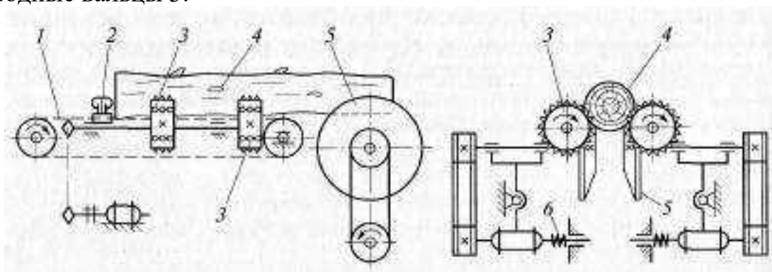
Рис. 9. Винтовой фрезерный окорочный станок:
