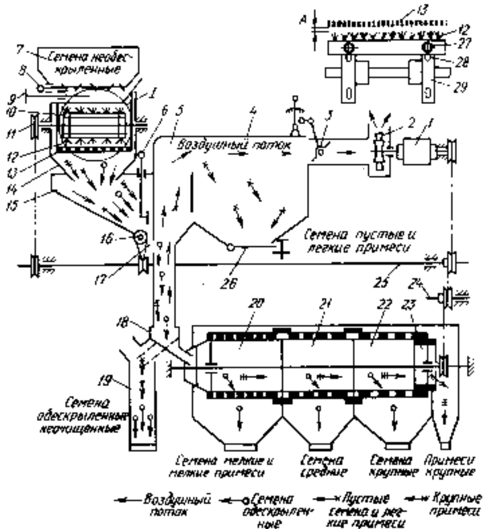
Рис. 14. Семяочистительная машина МОС-1:
