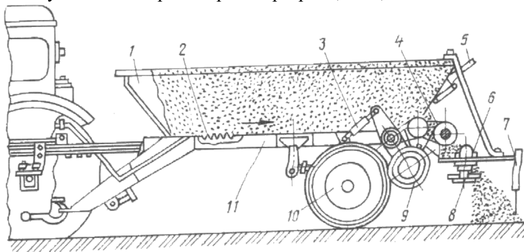
Рис. 15. Разбрасыватель минеральных удобрений 1-РМГ-4:
