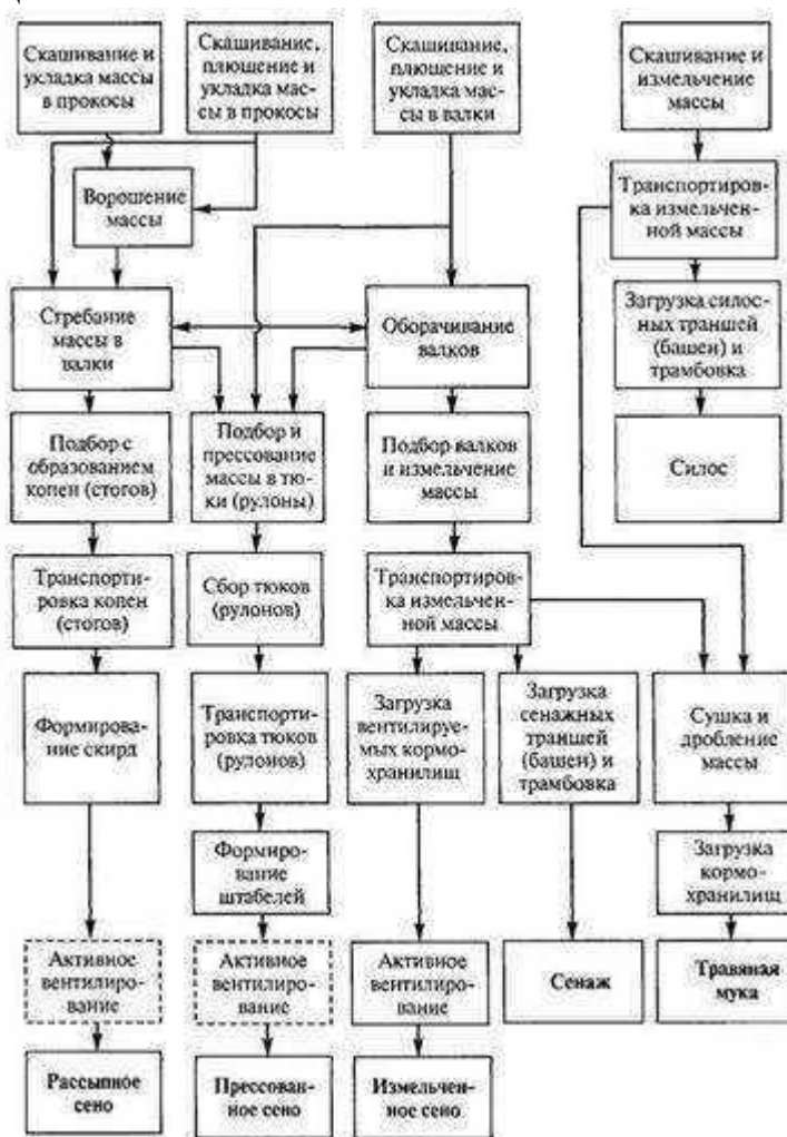
Рис.1.Схема технологий
