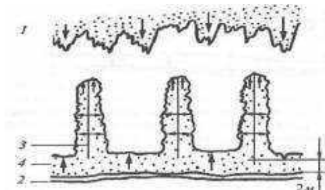
Рис.3. Отжиг способом «гребенки»: 1 - фронт пожара; 2 - опорная полоса; 3 - линия дополнительного зажигания; 4 - огонь отжига
