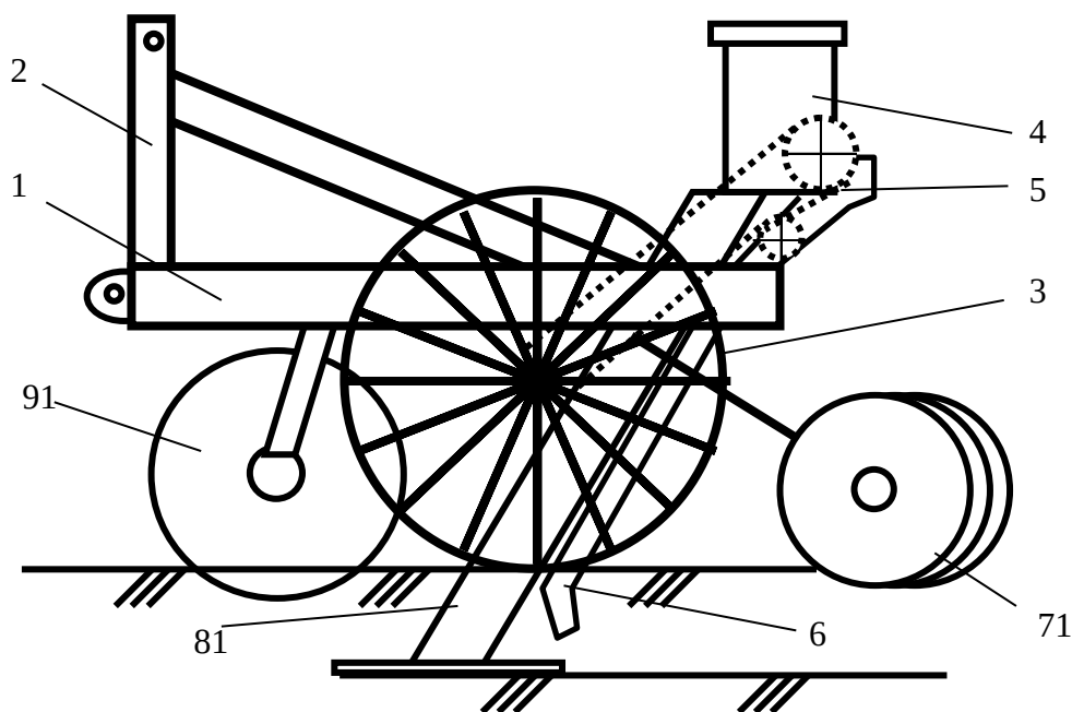
Рис. 2. Рыхлитель навесной РН-60:
