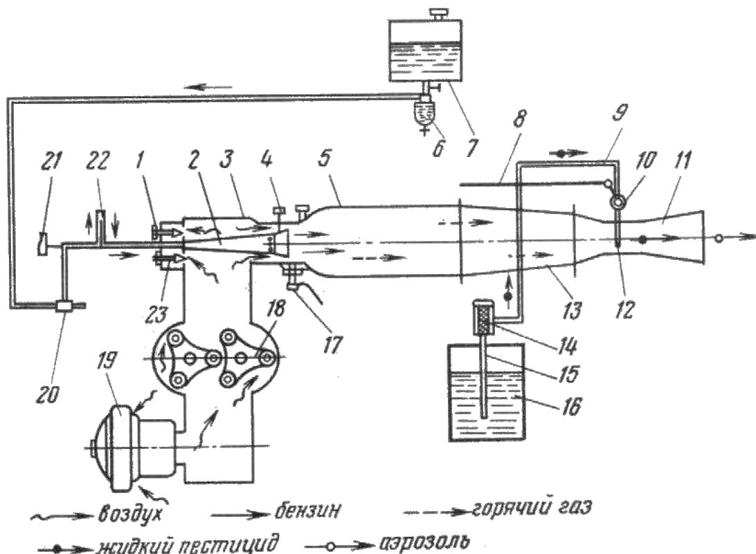
Рис. 17. Аэрозольный генератор АГ-УД-2:
