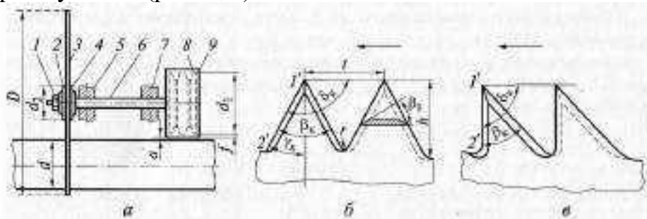
Рис. 2. Схема круглопильной установки для поперечной распиловки (а) и профили симметричных (б) и несимметричных (в) зубьев пильного
