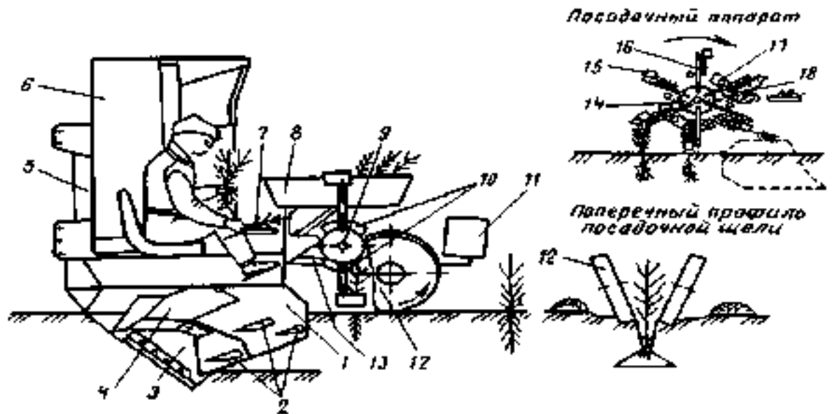
Рис. 11. Лесопосадочная машина МЛУ-1:
