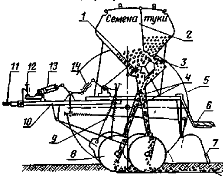
Рис. 12. Сеялка зернотуковая узкорядная СЗУ-3,6:
