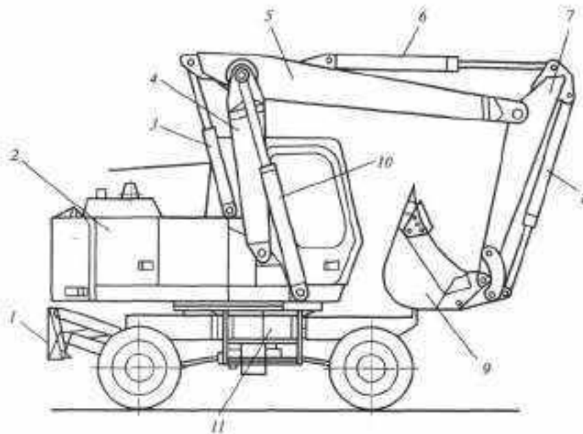
Рисунок 17. Одноковшовый полноповоротный экскаватор ЕК-12 с изменяемой геометрией рабочего оборудования:
