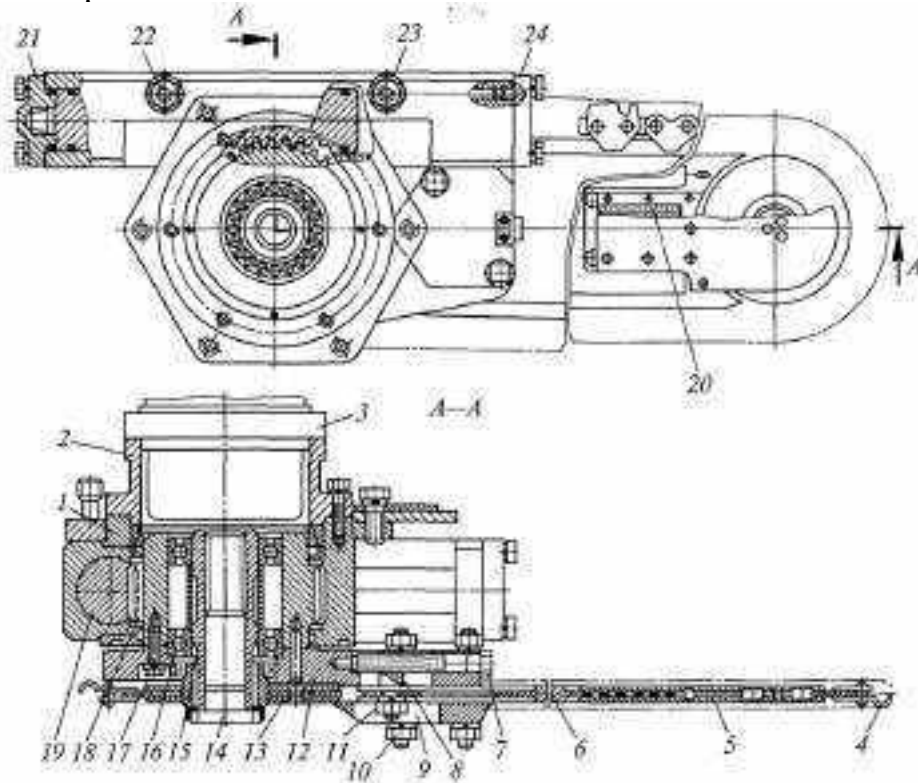
Рис. 3.6. Механизм срезания:
