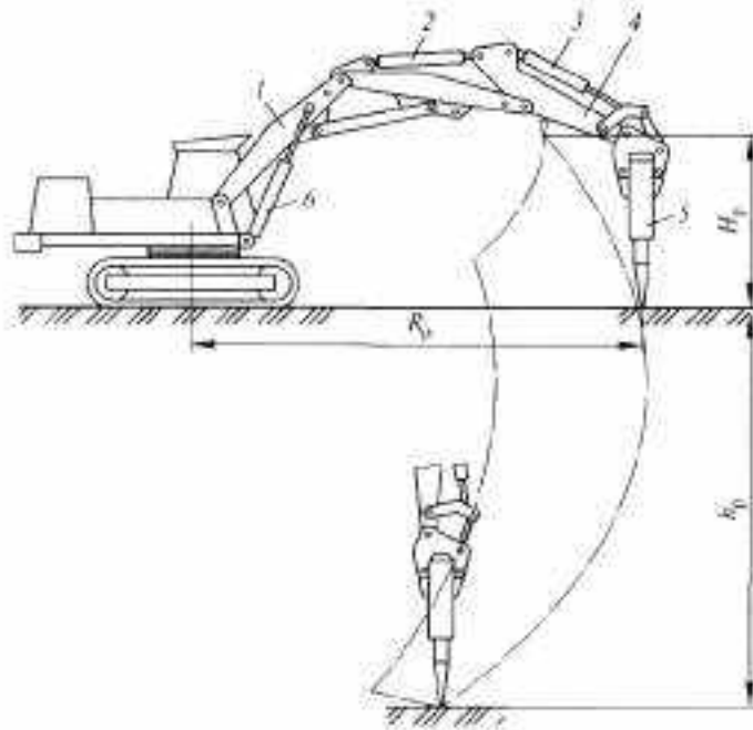
Рисунок 14. Экскаватор, оборудованный гидравлическим молотом
