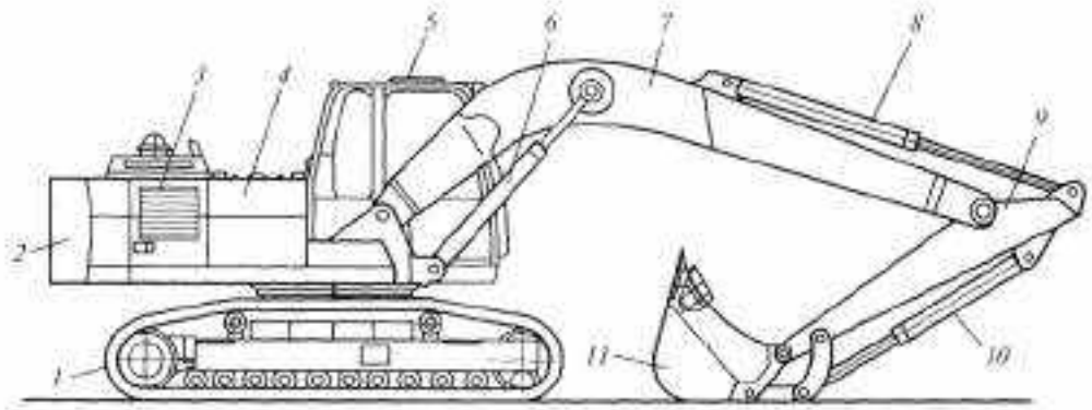
Рисунок 19. Одноковшовый полноповоротный гусеничный экскаватор ЕТ-18:
