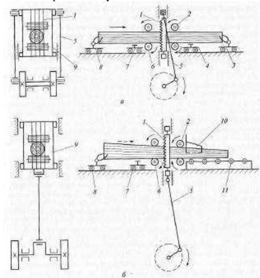
Рис. 6. Схемы двухшатунной (а) и одношатунной (б) лесопильных рам: 1 — пилы; 2, 6 — подающие валцы; 3, 4, 7, 8 — тележки; 5 — кривошипно-шатунный механизм; 9 — пильная рамка; 10 — направляющий нож; 11 — рольганг
