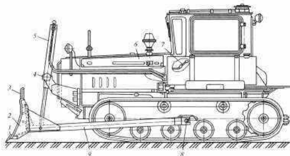
Рис. 4.9. Бульдозер Д3-42F
