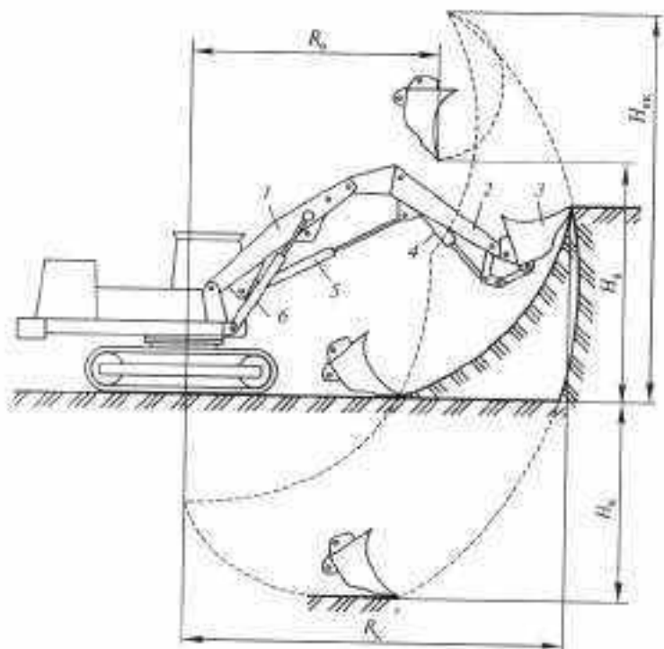
Рисунок 10. Экскаватор с рабочим оборудованием прямая лопата
