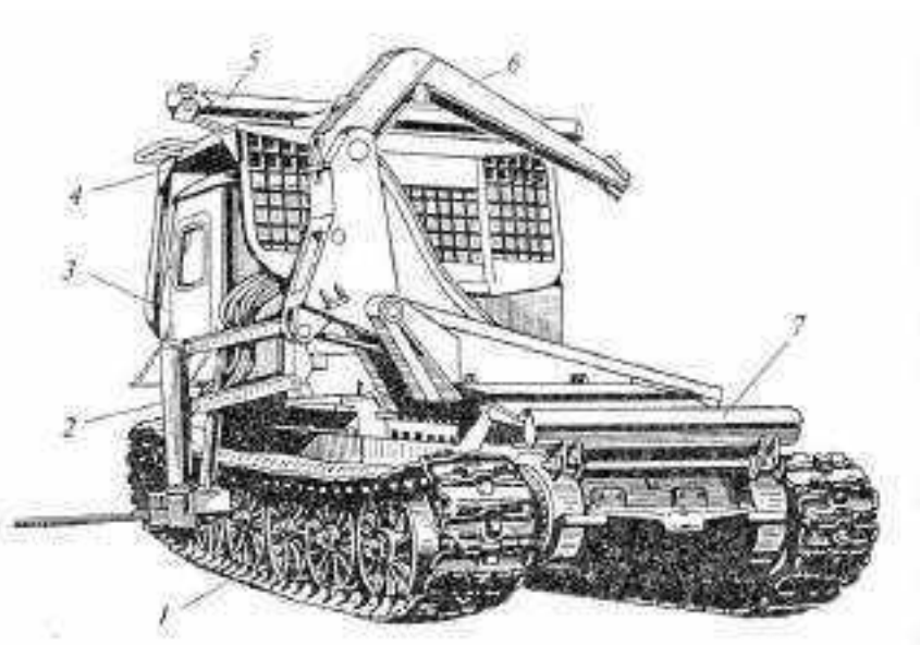
Рис. 3.1. Валочная машина ВМ-4.
