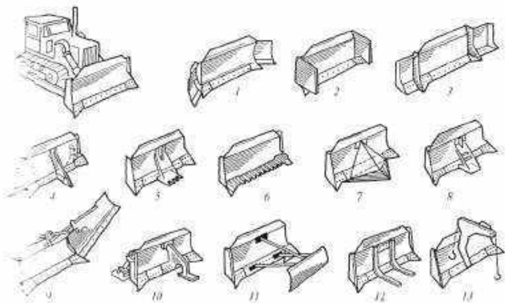
Рис. 4.8. Сменные рабочие органы гусеничных бульдозеров
