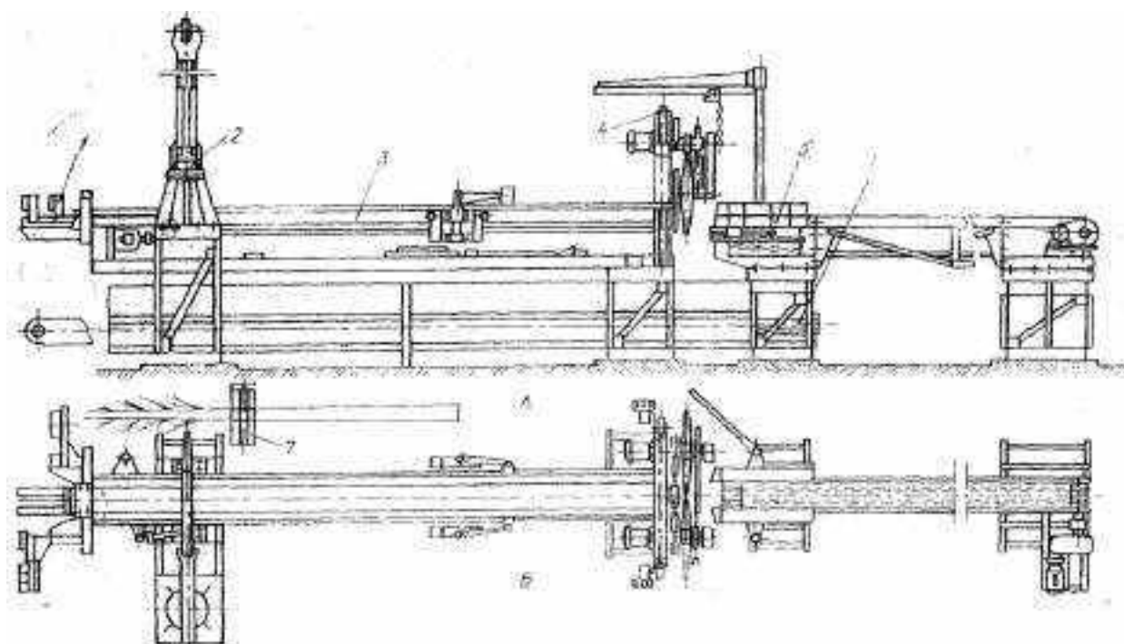
Рис. 2. Сучкорезно-раскряжеочная установка ЛО-30:
