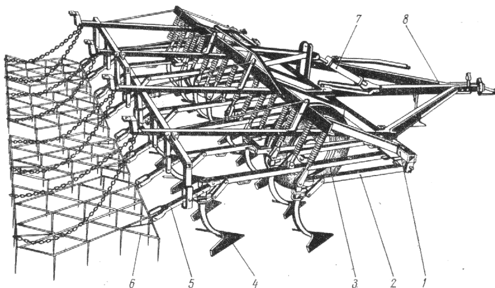
Рис. 9. Культиватор КПС-4 с зубовыми боронами:
