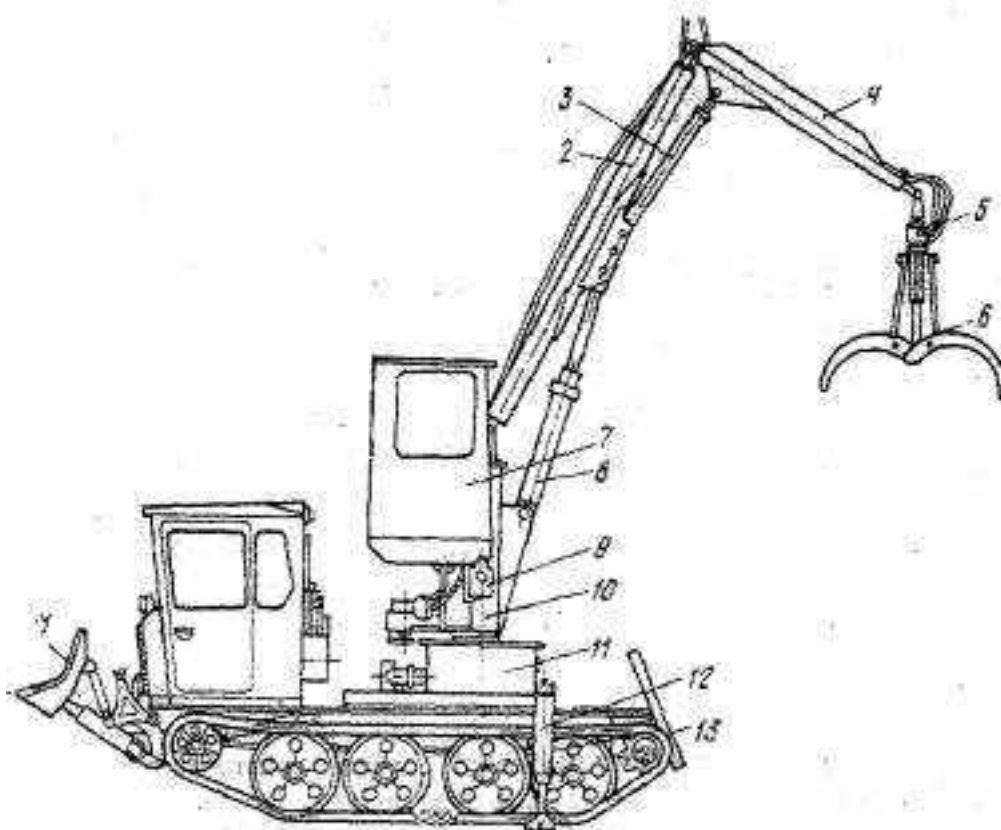
Рис. 4. Погрузчик-штабелер ПШ-80:
