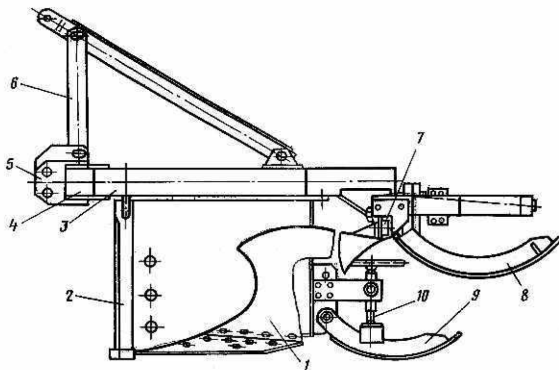
Рис. 1. Плуг лесной ПЛ-1:
