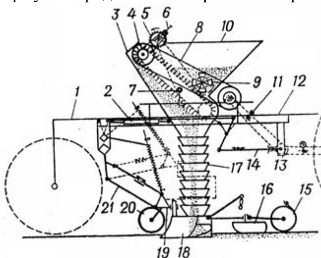
1- самоходное шасси; 2- гидроцилиндр; 3- семяприемник; 4- транспортер; 5- щеточный ограничитель; 6- регулировочный винт; 7- натяжной ролик; 8- клиноременная передача; 9- ворошилка; 10- бункер; 11- натяжное устройство; 12- рама; 13- муфта; 14- тяга; 15- прикатывающий каток; 16- загортач; 17- семяпровод; 18- сошник; 19- кронштейн; 20- опорное колесо; 21- рама с механизмом подъема секции.
