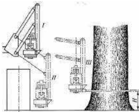
Рис. 1.3. Положение вертикальной наводки механизма срезания: I — транспортное; II — предельно нижнее; III — рабочее при высоте пня; H — высота пня
