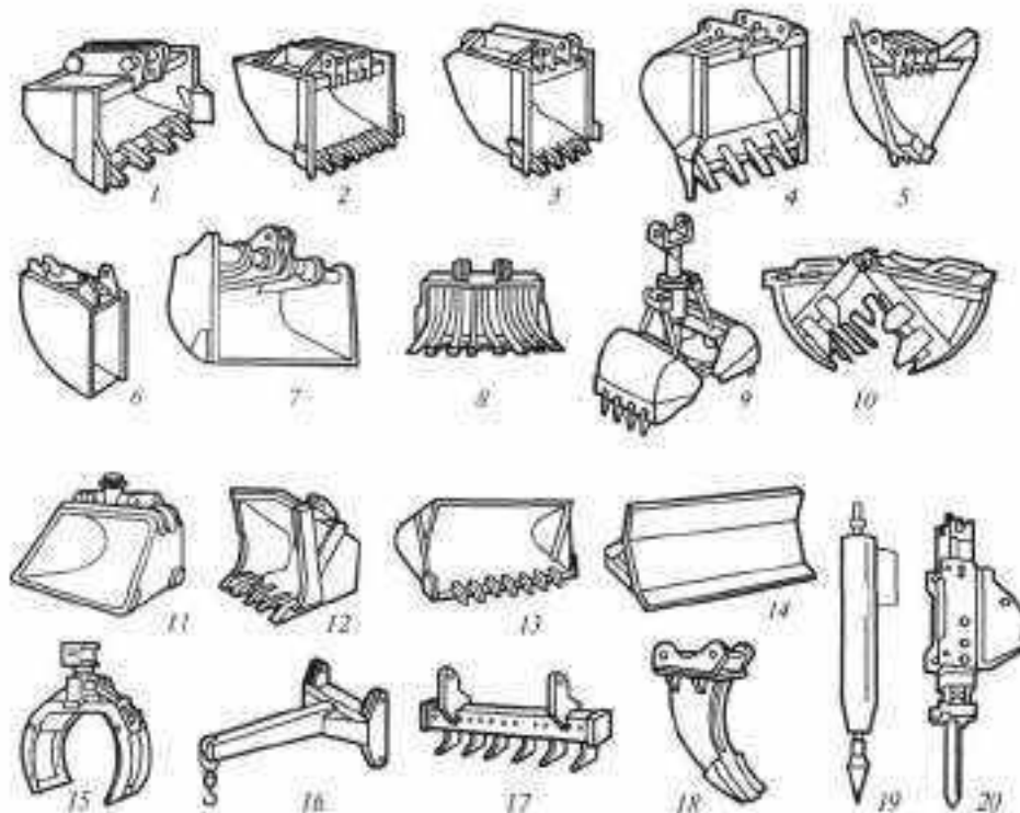
Рисунок 8. Сменные рабочие органы гидравлических экскаваторов
