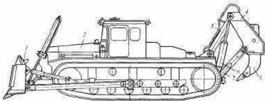
Рис. 4.1. Бульдозер-рыхлитель ДЭТ-250М2Б1Р1
