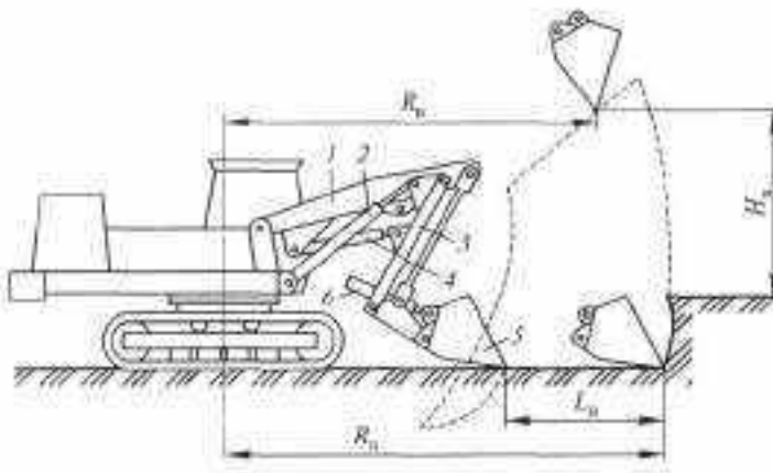
Рисунок 11. Экскаватор с погрузочным оборудованием
