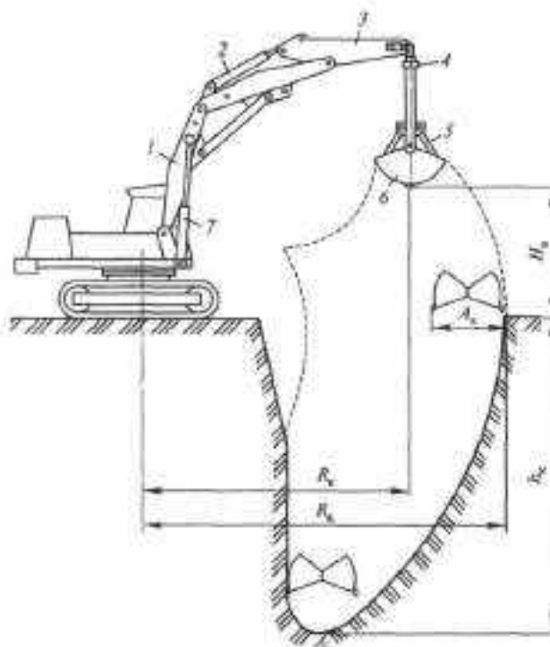
Рисунок 12. Экскаватор с грейферным оборудованием
