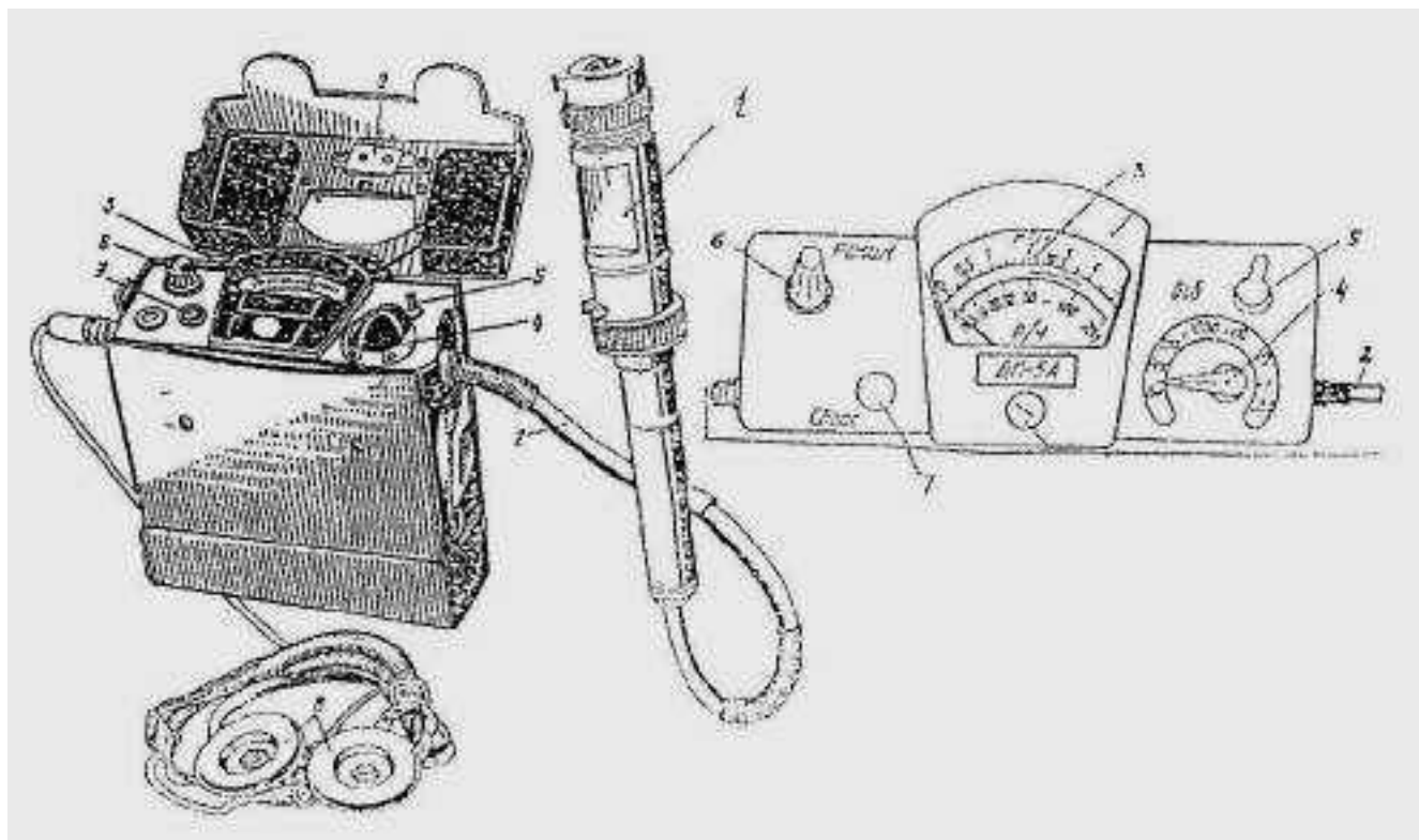
Рис. 1. Рентгенометр ДП - 5А
