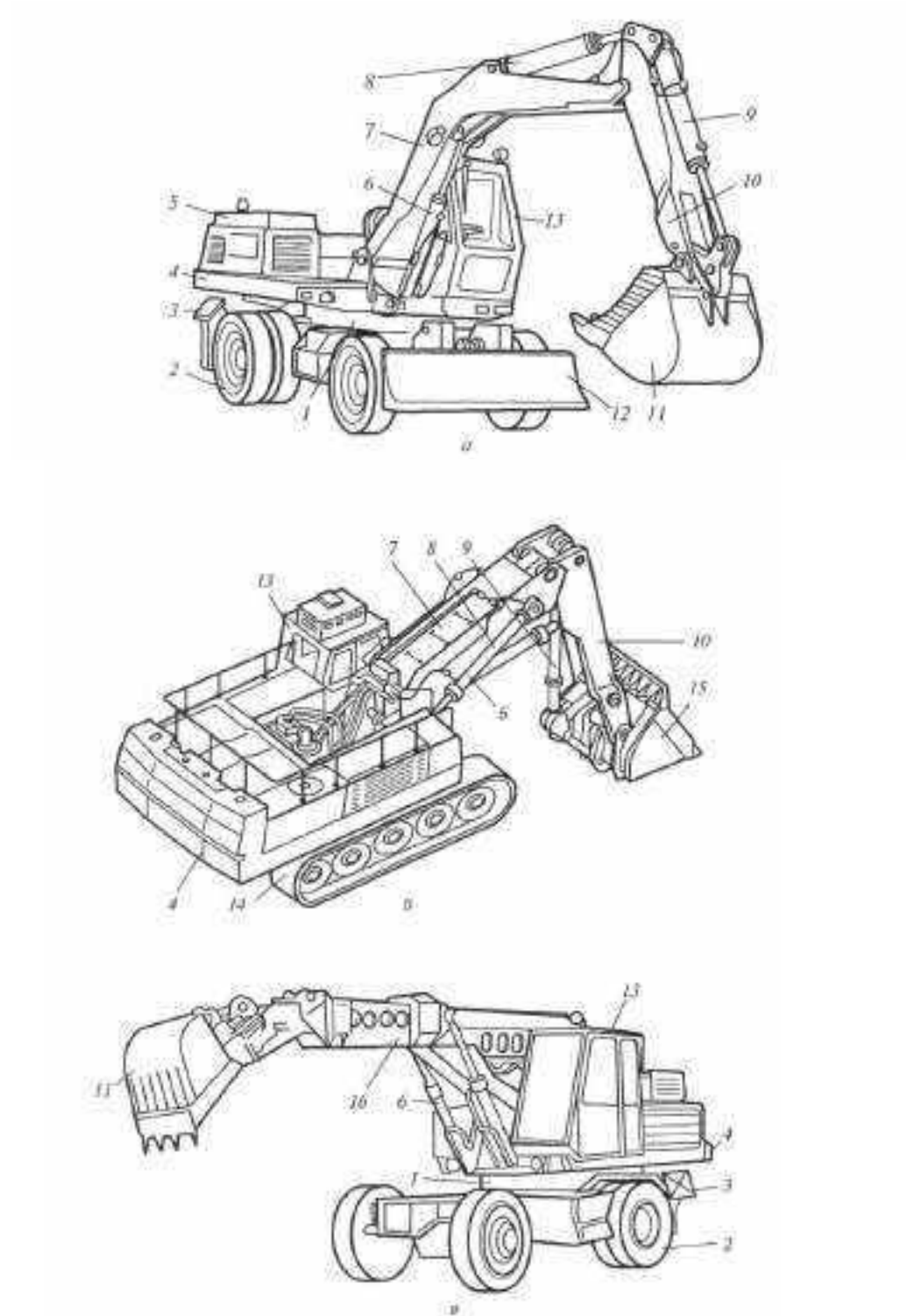
Рисунок 7. - Одноковшовые гидравлические полноповоротные экскаваторы с жесткой подвеской рабочего оборудования:
