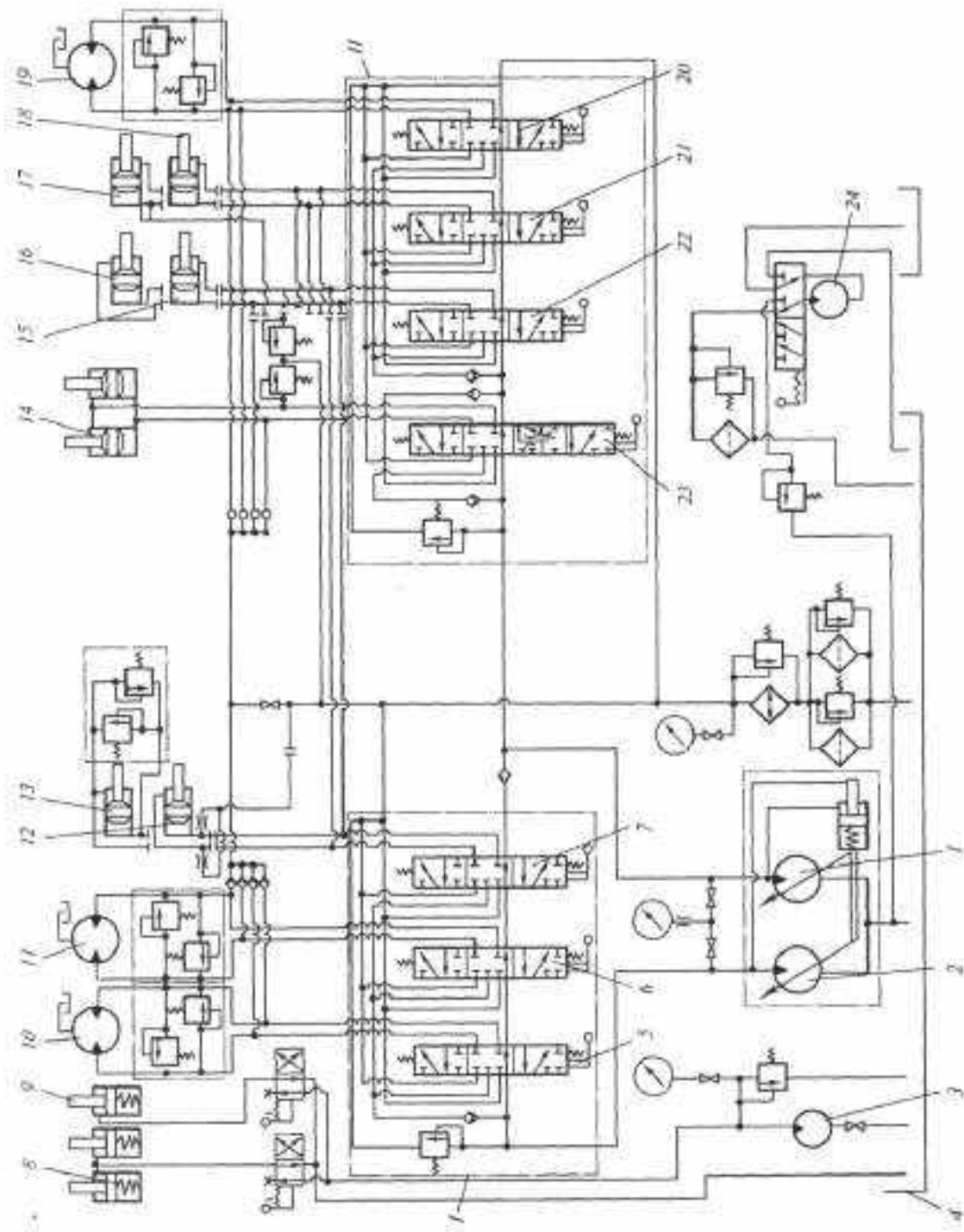
Рис. 4.41. Типовая гидравлическая схема полноповоротных экскаваторов четвертой размерной группы
