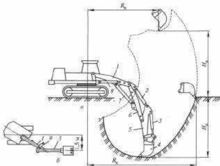
Рисунок 9 . Экскаватор с рабочим оборудованием обратная лопата
