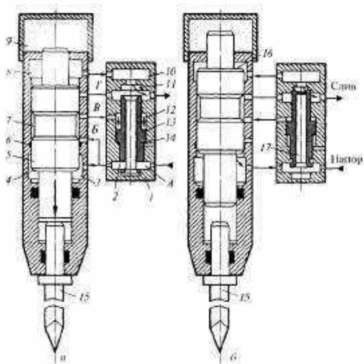
Рисунок 16. Принципиальная схема гидropневматического молота
