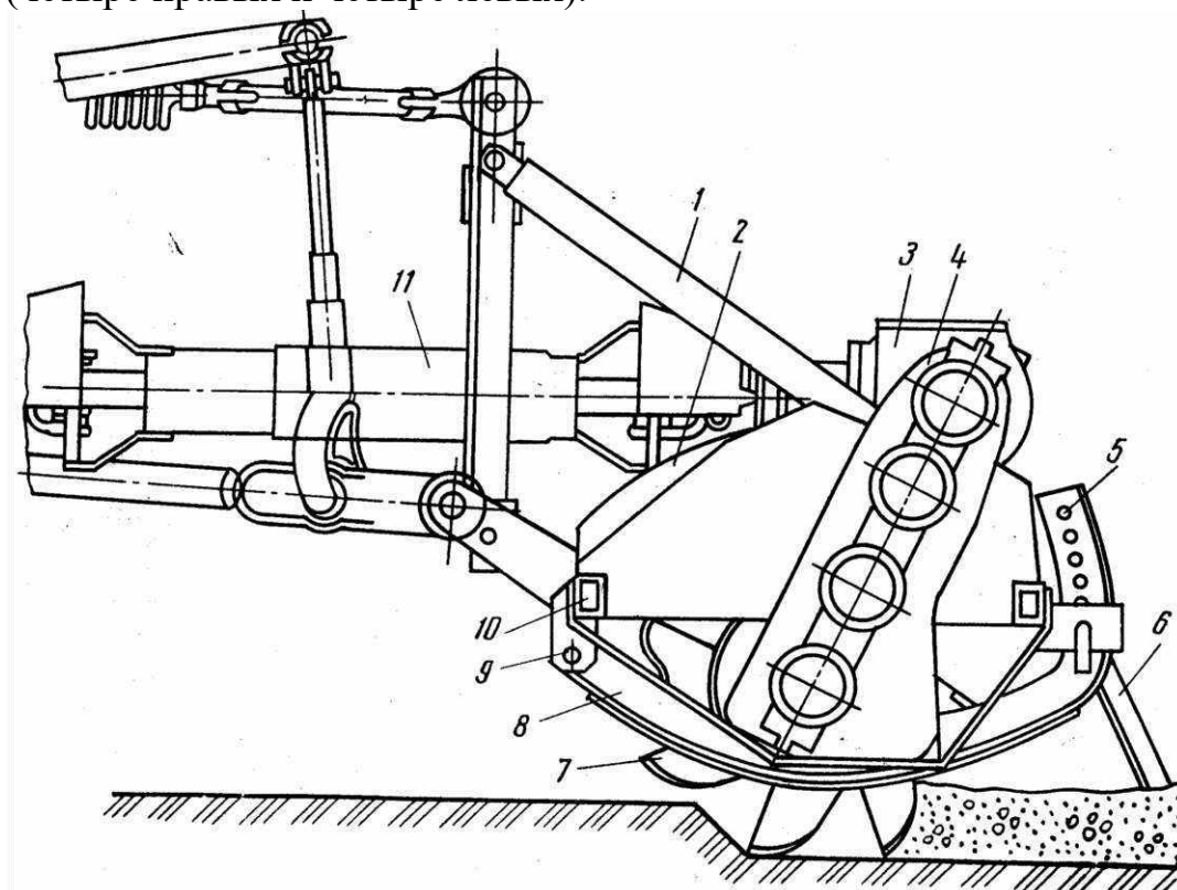
Рис. 5. Фреза лесная унифицированная ФЛУ-0,8:
