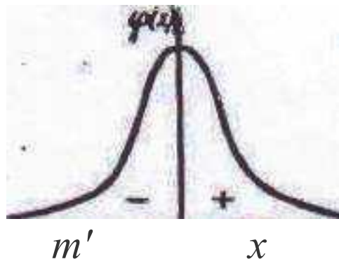
Рис. 17. Кривая плотности вероятности нормально распределенной случайной величины: x — среднее значение; \phi(x) — относительная вероятность измерения x
