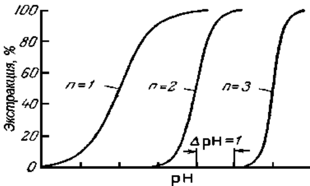
Рис.11.Кривые экстракции
