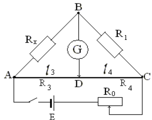
Рис.2 Схема мостика Уитстона
