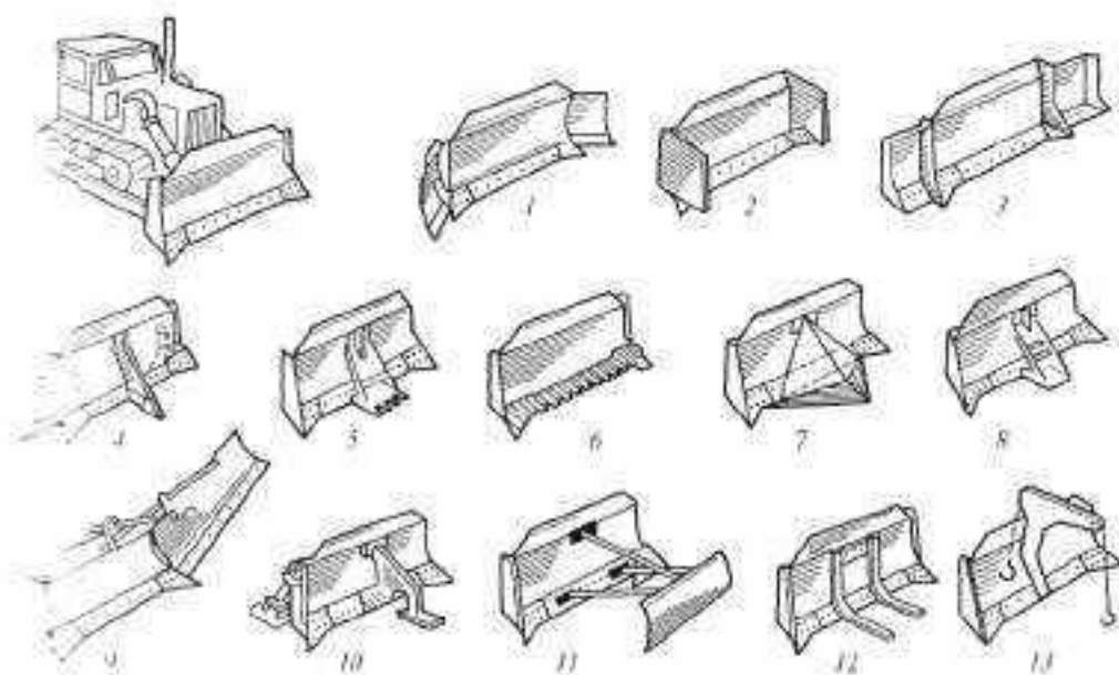
Рис. 4.8. Сменные рабочие органы гусеничных бульдозеров.
