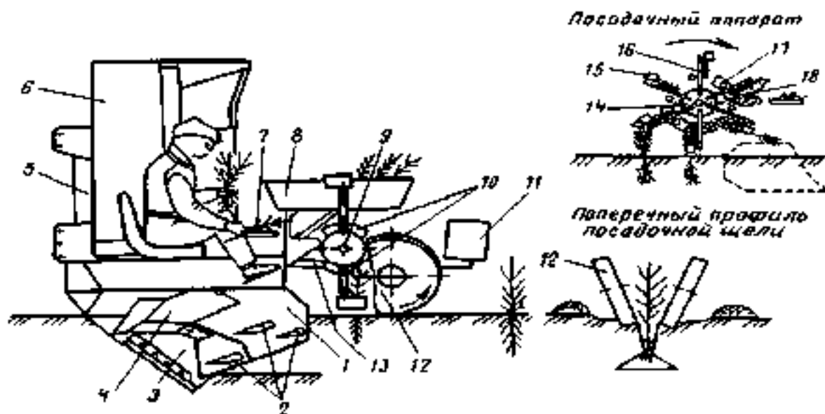
Рис. 11. Лесопосадочная машина МЛУ-1:
