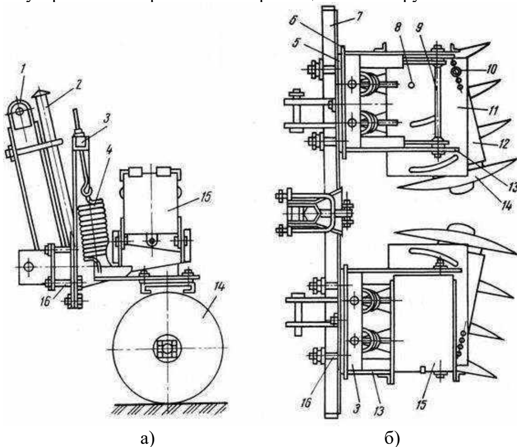
Рис.7. Культиватор лесной бороздной КЛБ-1,7:
