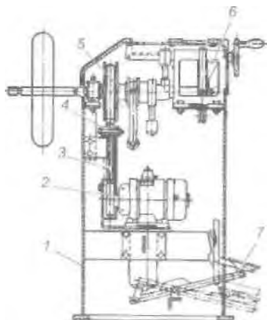
Рис. 3. Балансировочный станок для колес легковых автомобилей: / — корпус; 2 — электродвигатель; 3 — ременная передача; 4 — тормозное устройство; 5 — балансировочный механизм; 6 — резонансный индикатор; 7 — педаль
