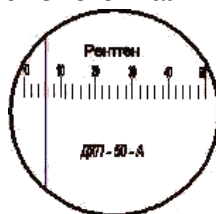
Рисунок 11 Дозиметр карманный прямопоказывающий ДКП-50А
